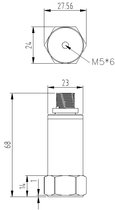
图 3 产品外形及安装尺寸图
