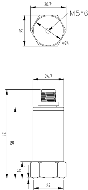
图 3 产品外形及安装尺寸图
