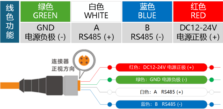
图 2 传感器信号线对应色标
